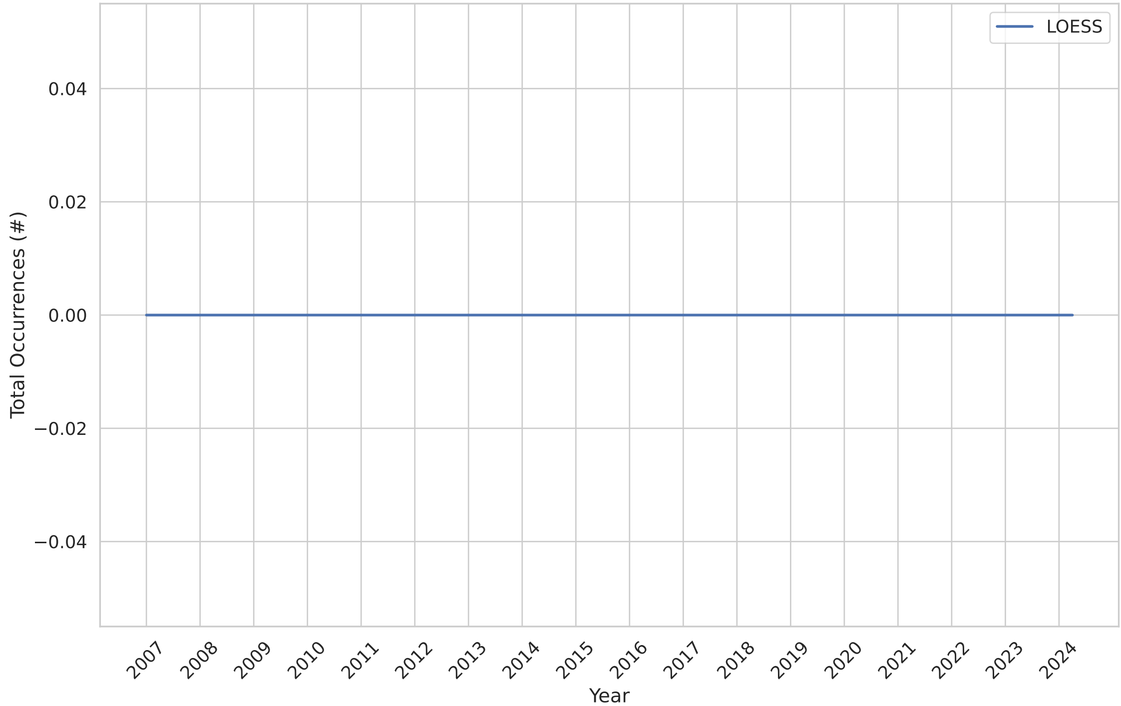
Type Parameter Syntax — Trend
